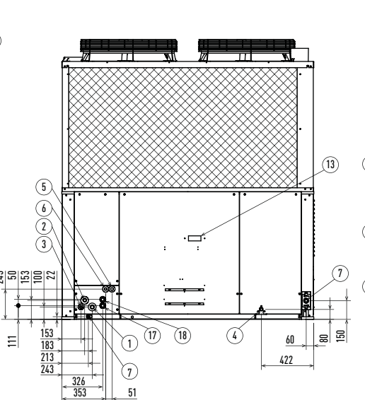
Rückansicht
