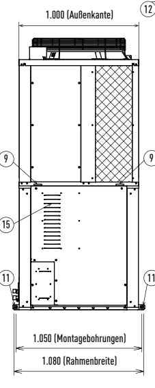
Seitenansicht links
