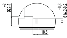
Detailsicht B
