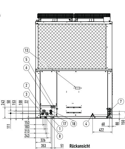
Rückansicht
