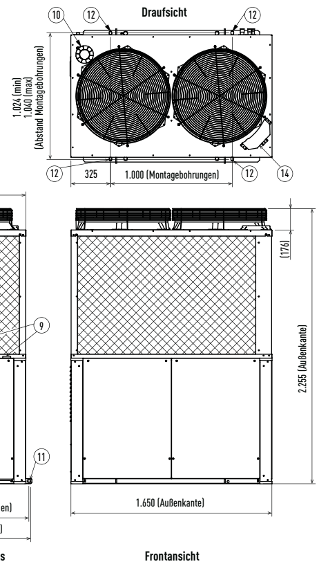
Frontansicht
