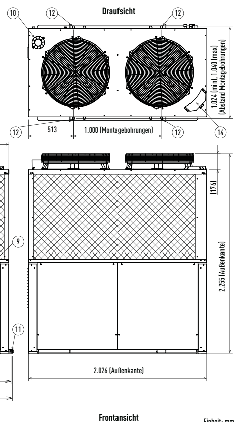
Frontansicht
