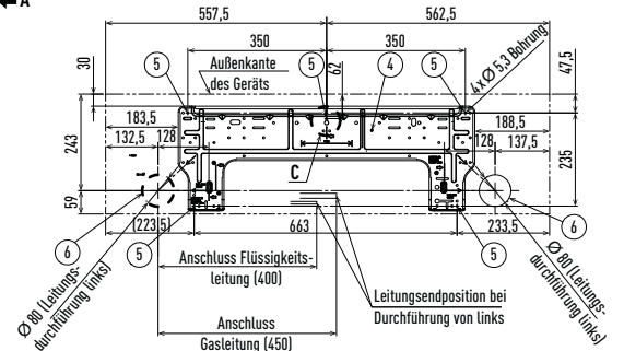
Ansicht A
