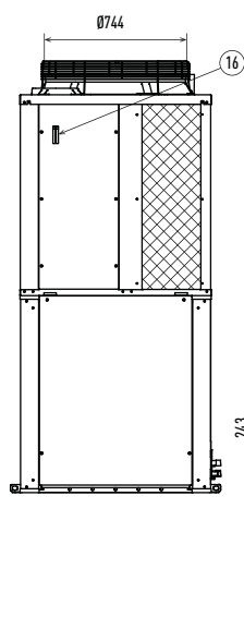
Seitenansicht rechts
