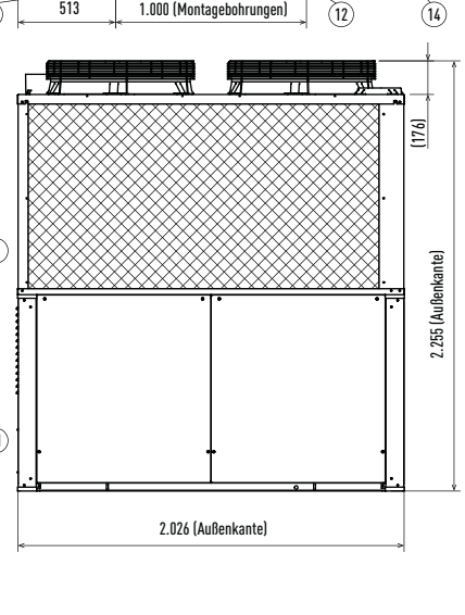
Frontansicht
