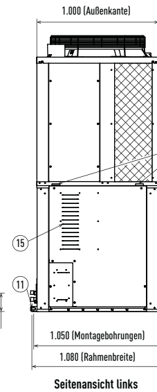
Seitenansicht links
