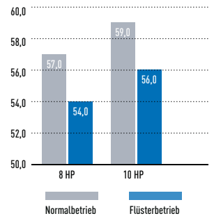
Schalldruckpegel (dB(A))
