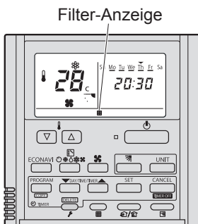
Timer-Fernbedienung
