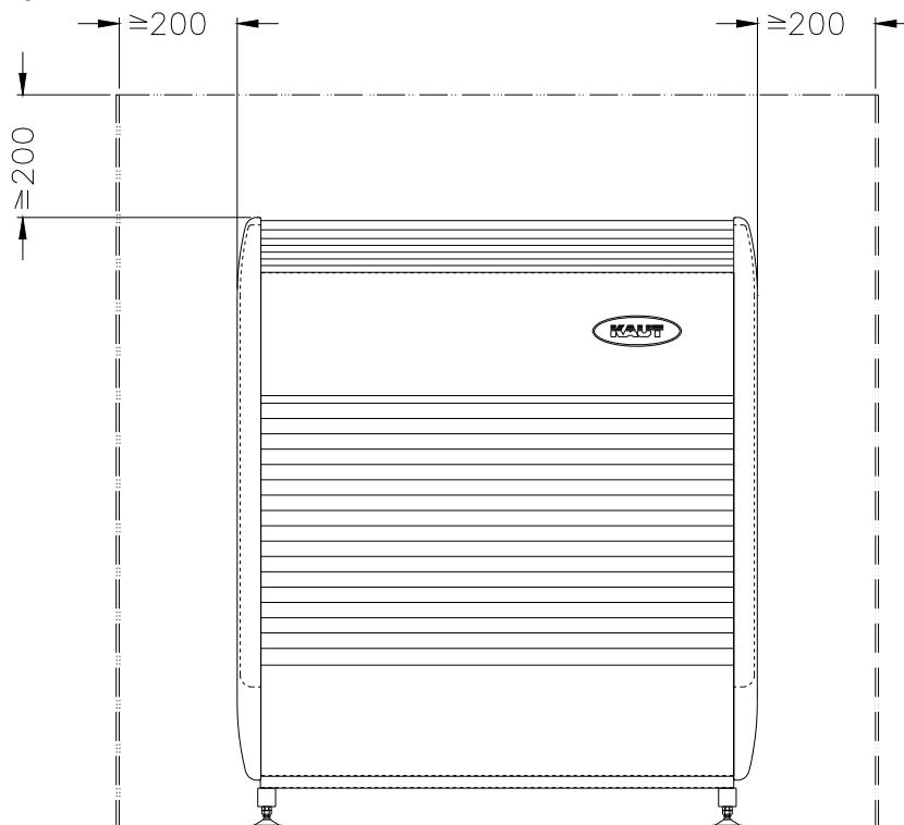
Abb.1: einzuhaltende Abstände
