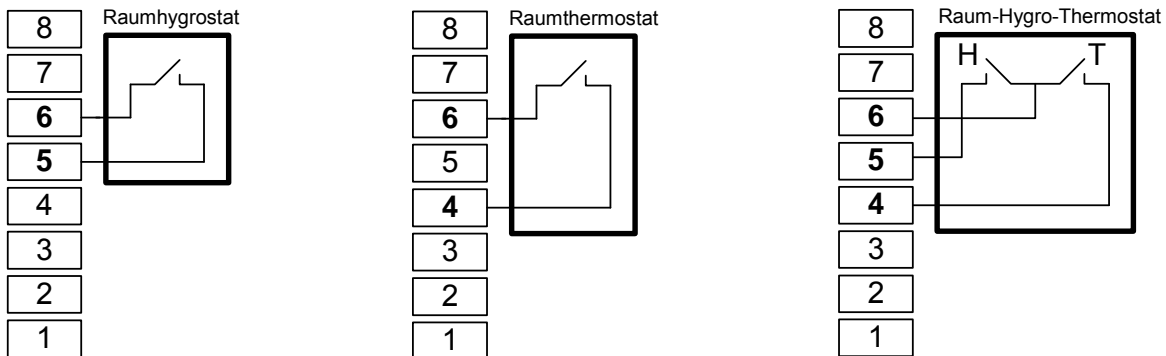
Abb.: 5.1 Klemmenbelegung und Anschluss externer Steuergeräte (Zubehör)
