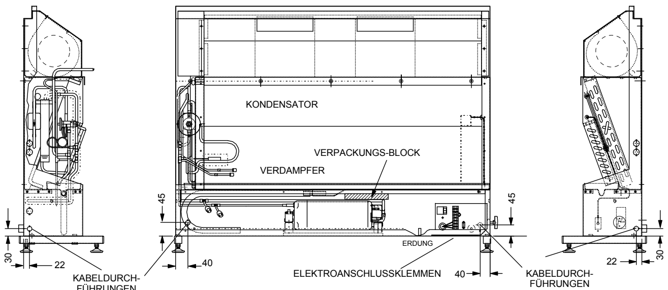
Abb. 5: Position der Kabeldurchführungen und Anschlussklemmen
