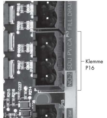
ABBILDUNG 24-1: KLEMME P16
