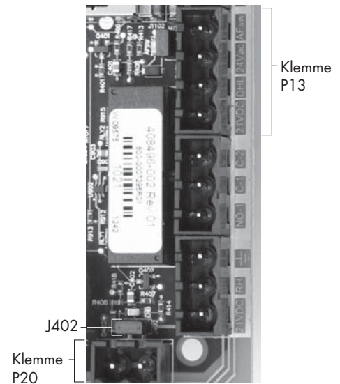
ABBILDUNG 16-1: KLEMME P13
