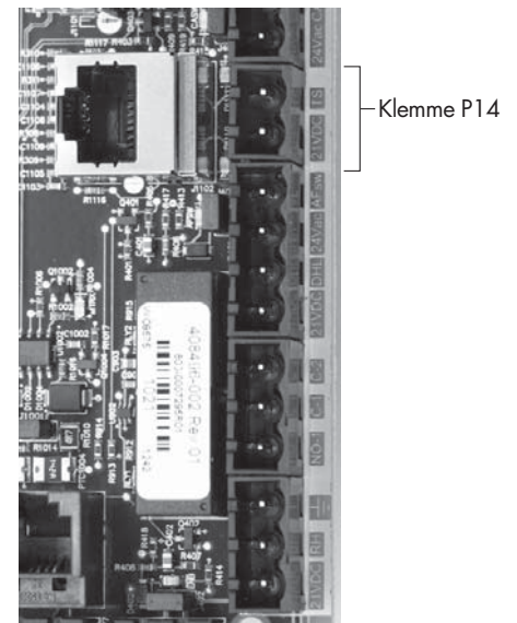
ABBILDUNG 18-1: KLEMME P14
