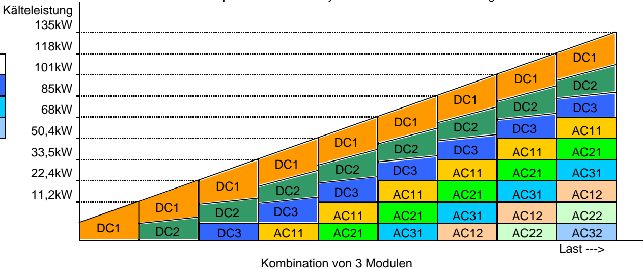
Beispiel ECO-i 3WAY System mit 135kW Kälteleistung
