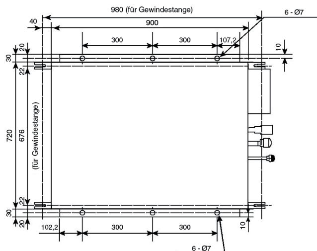
DRAUFSICHT
