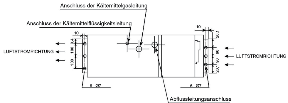
DRAUFSICHT
